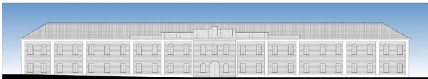
VERBOUWEN VOORMALIG KAZERNEGEBOUW TOT CENTRUM VOOR VEILIGHEIDSDIENSTEN POLITIEKANTOOR 'ZONE GRENSLEIE' - BRANDWEERKAZERNE - RODE KRUIS - CIVIELE BESCHERMING GEVELAANZICHT LEOPOLDPLEIN
